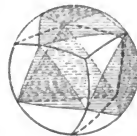
Fig. 16. Tetraedroid.
